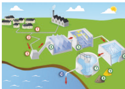
Schéma d'un système d'assainissement collectif.
